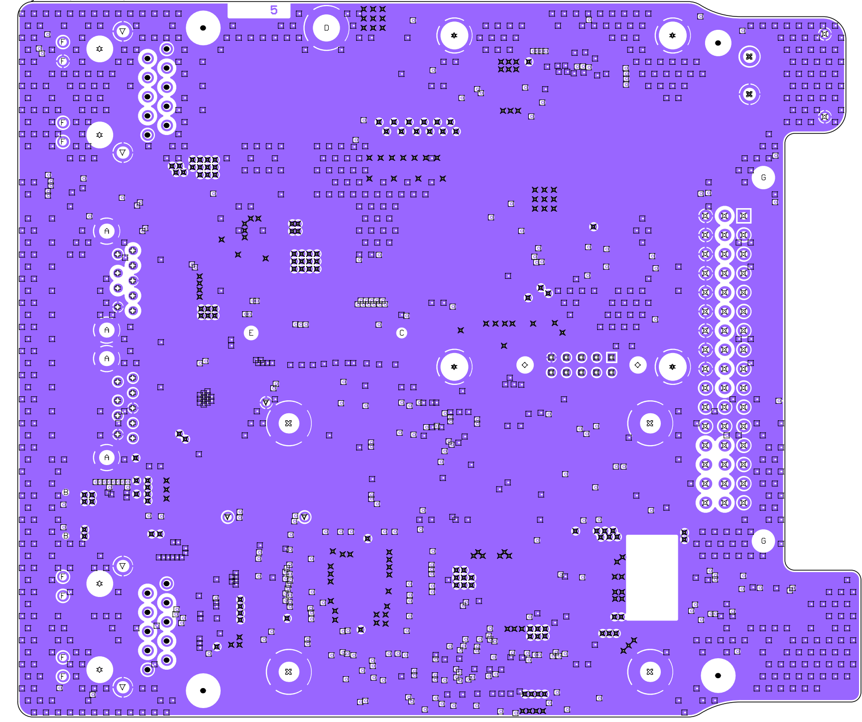
Layer 5 (Scale 2:1)
