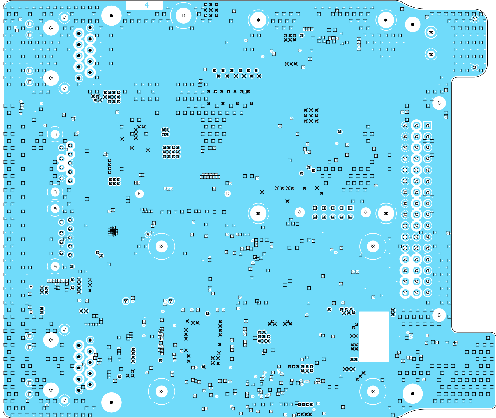
Layer 4 (Scale 2:1)
